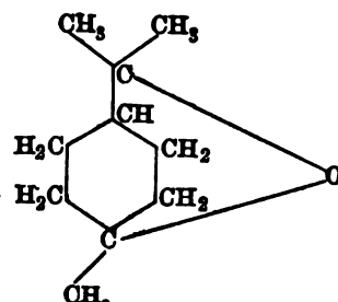
Cineol, eucalyptol .
